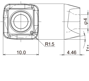
Fig.2 SPET100415ZPER-SM
